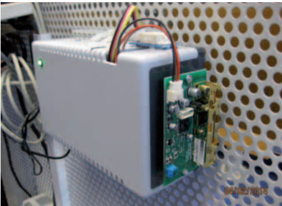
Abbildung 1: Messeinheit für Luftgüte und Lautstärke
