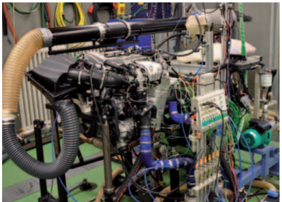
Der Versuchsmotor der Adam Opel AG mit allen Messinstrumenten im Motorenlabor des Instituts für Fahrzeugtechnik (ift) der Hochschule Trier.
